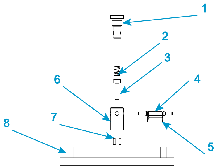
图 17.O 型底座联接头
