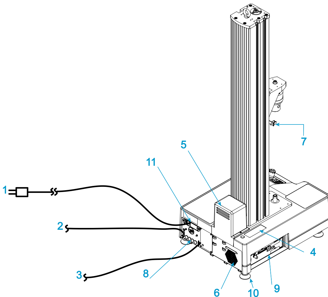
图 5. 机架连接
